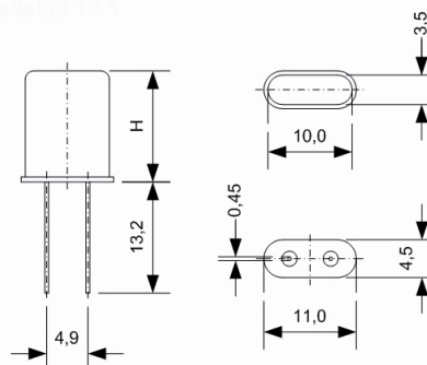
Meßtab 1:1
